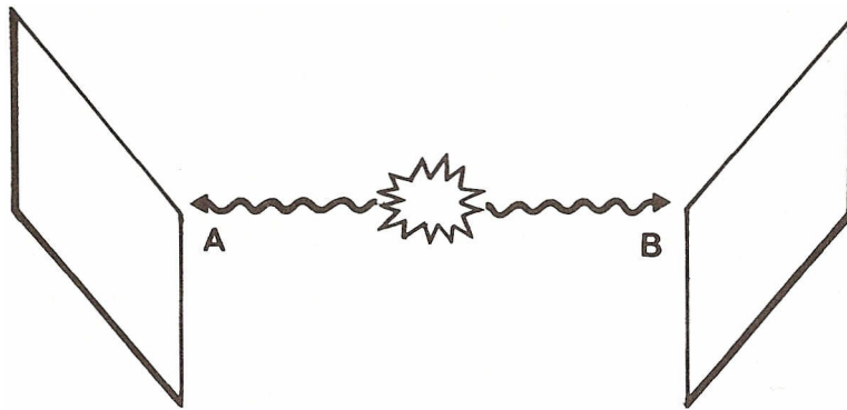
Fig. 13. Contrastación de la desigualdad de Bell: Si los polarizadores se orientan oblicuamente, la cooperación entre A y B se reduce; a veces A pasa y B queda bloqueado. Sin embargo, algo de cooperación queda. En particular, hay más cooperación de la que puede explicar una teoría que a) acepte la realidad independiente del mundo externo y b) niegue la existencia de comunicación hacia el pasado entre los distantes fotones.
