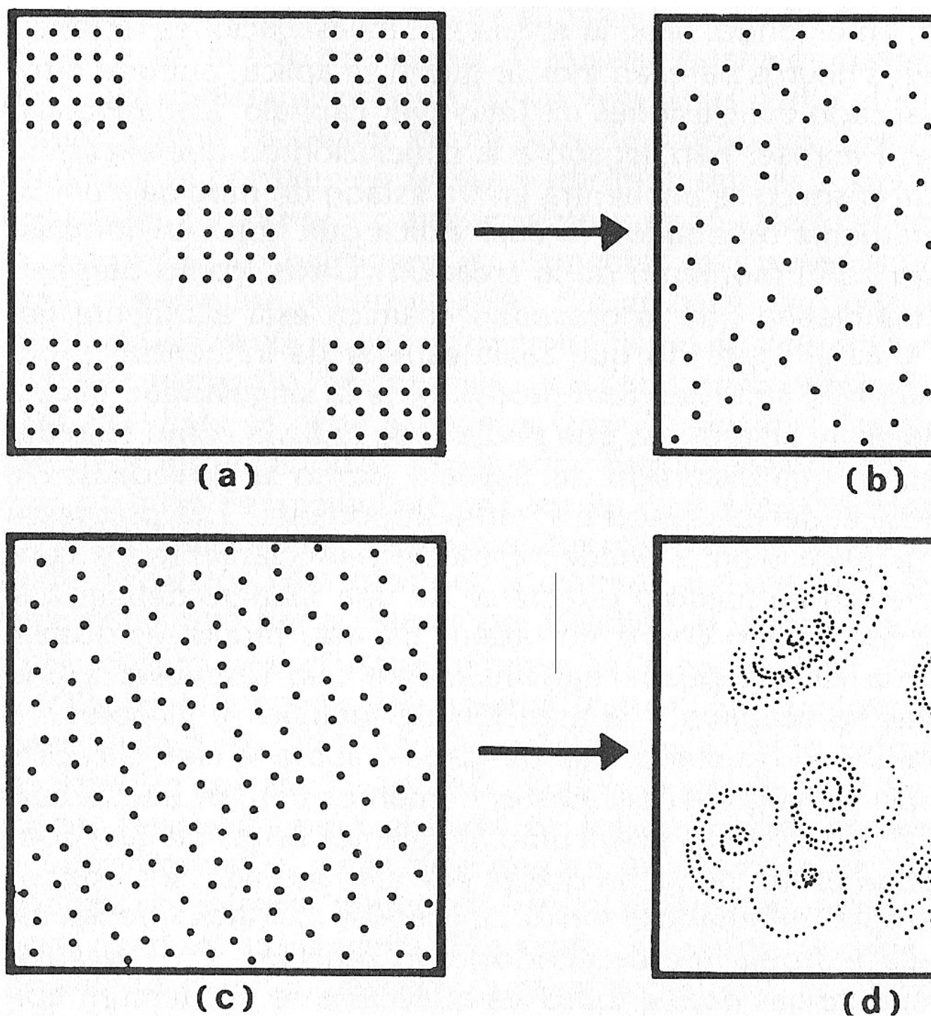
Fig. 7. El concepto de orden depende crucialmente de si podemos o no ignorar la gravedad. El recuadro (a) contiene un gas para el que la gravedad es negligible. Su ordenada disposición molecular pronto se transforma en desorden amorfo (máxima entropía) a causa de las colisiones entre moléculas. El estado final es (b). Por otra parte, un "gas" gravitante —un sistema estelar, por
