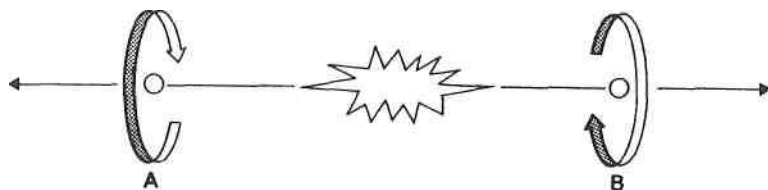
Fig. 11. La desintegración de un átomo o de una partícula subnuclear puede dar lugar a dos partículas
