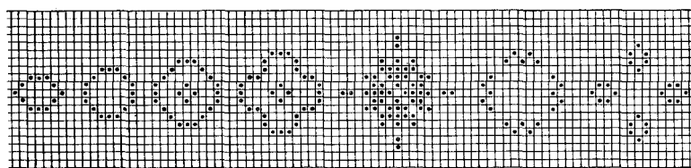
Fig. 25. En el juego de la vida de John Conway, la sucesión de estructuras de la figura evoluciona (hemos omitido algunos pasos intermedios). Las formas son reminiscentes del ciclo vital de una flor.
